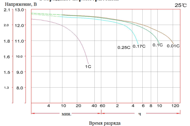
Разрядные характеристики
